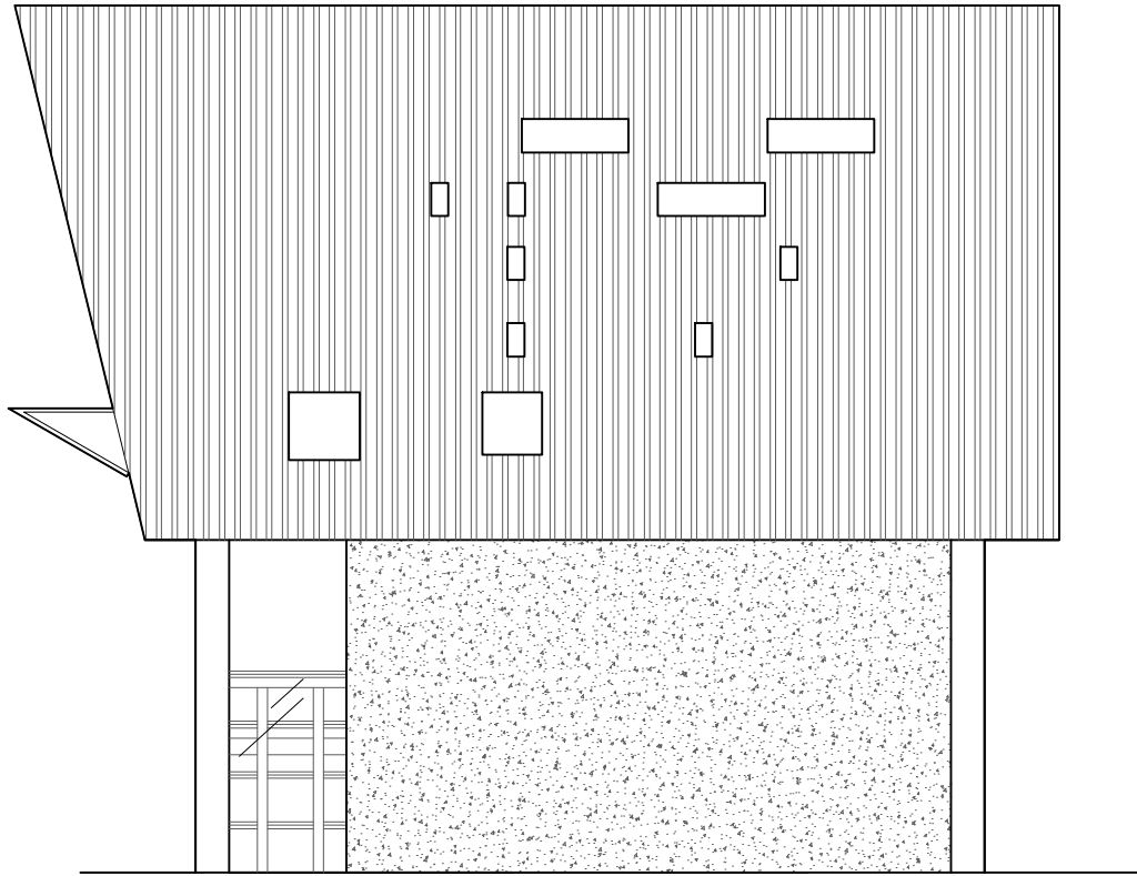
1 TAMPAK SAMPING KANAN SKALA 1:50
