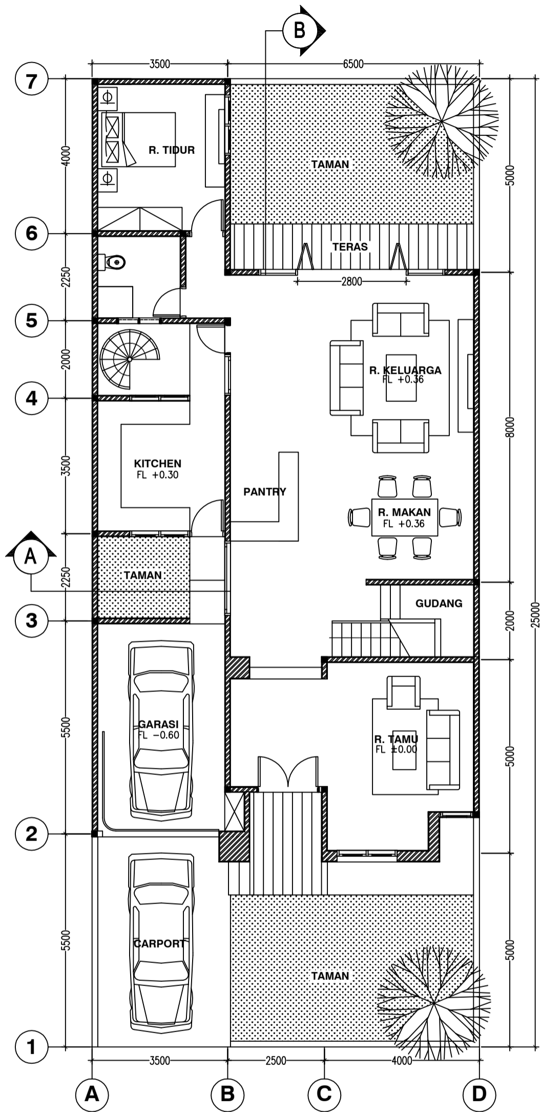
DENAH LT BAWAH 1 : 100
